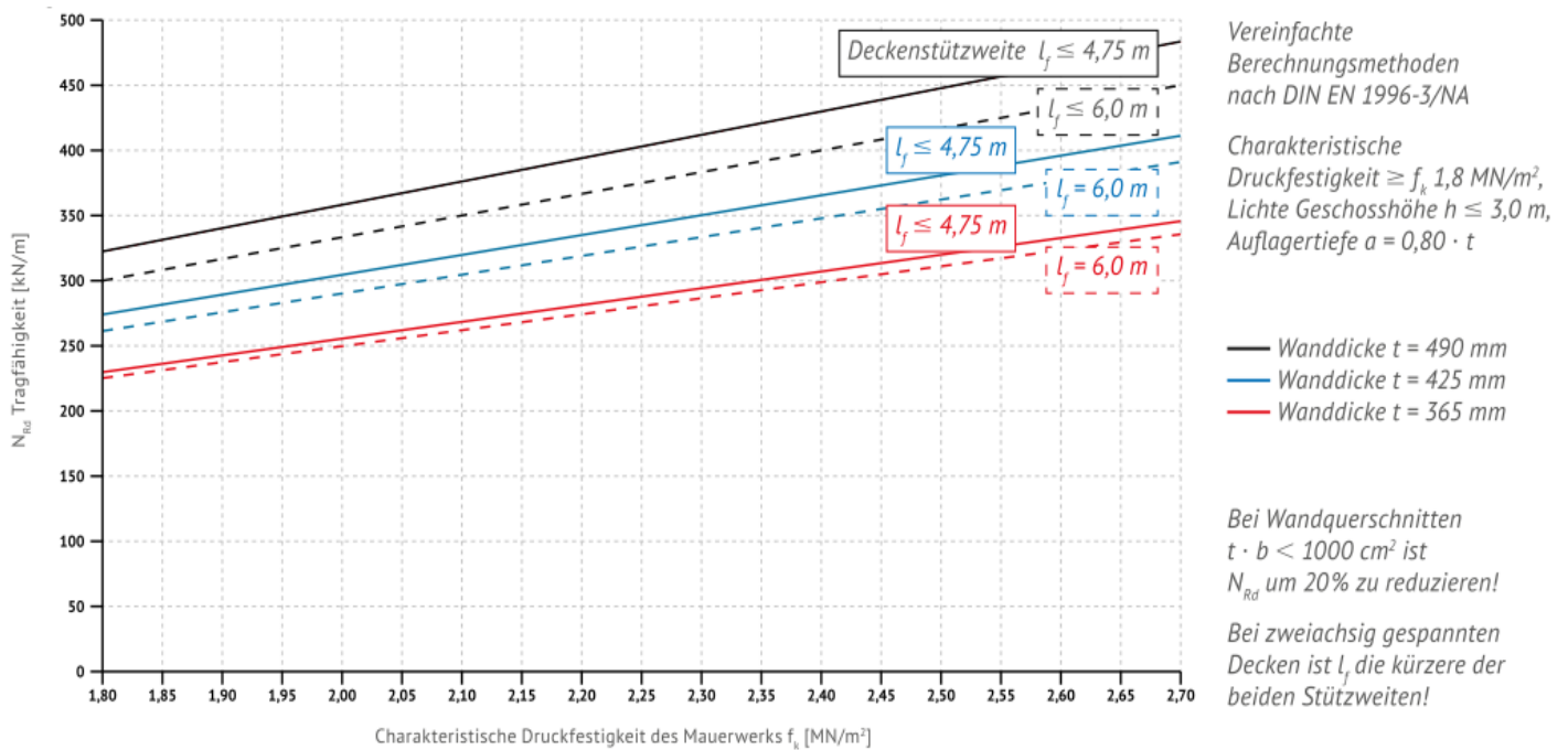
Diagramm 2. Tragfähigkeit N_{Rd} [kN/m] von Bisotherm Außenwänden ( a/t = 0,80 ; f_k \geq 1,8 \text{ MN/m}^2 )
