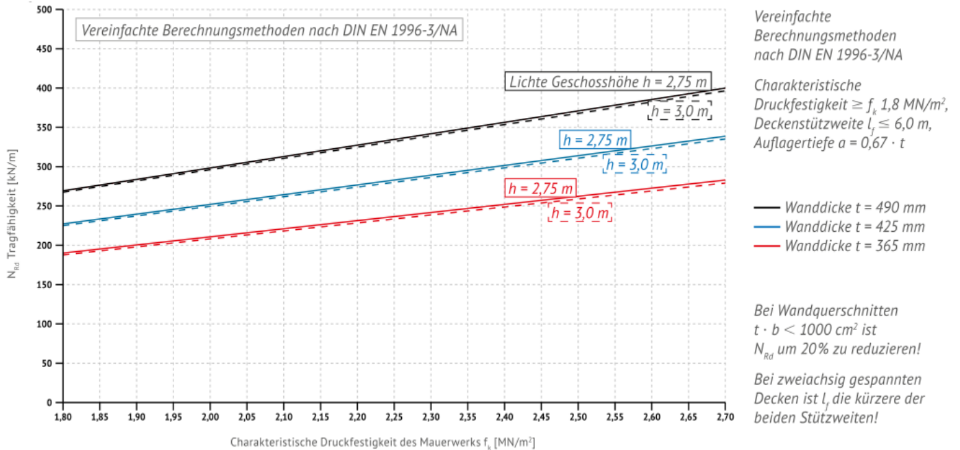
Diagramm 1. Tragfähigkeit N_{Rd} [kN/m] von Bisotherm Außenwänden ( a/t = 0,67 ; f_k \geq 1,8 \text{ MN/m}^2 )
